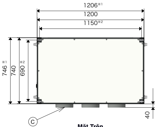
Mặt Trên
