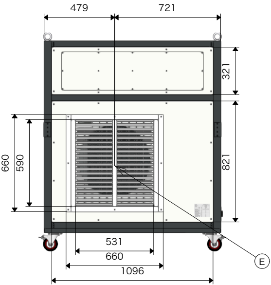
Mặt Sau
