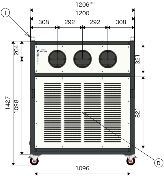
Mặt Trước
